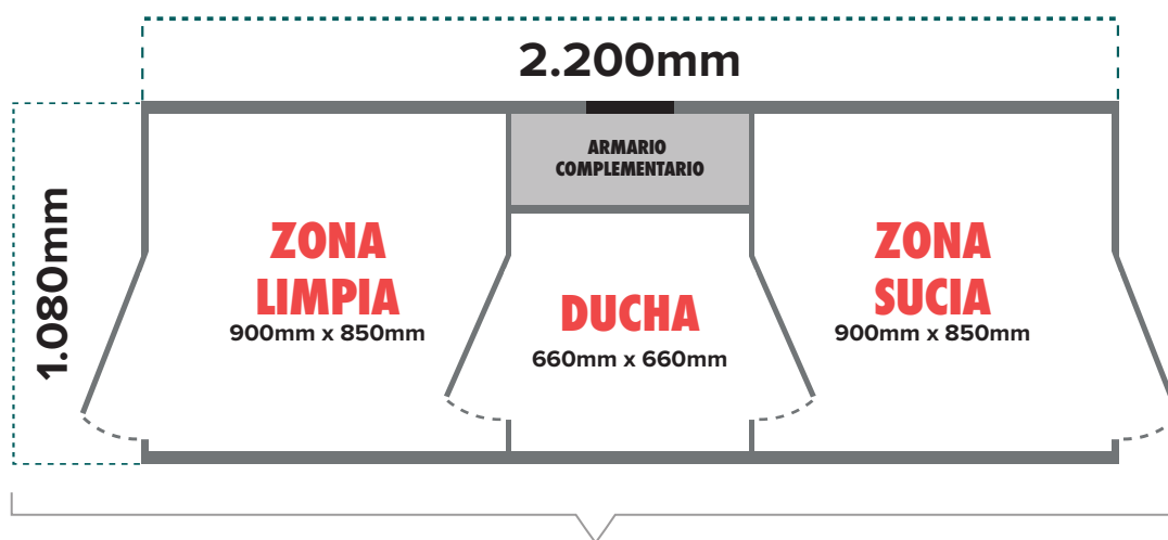
Plano a escala de U.M.D. Modelo: BASE 220/10
