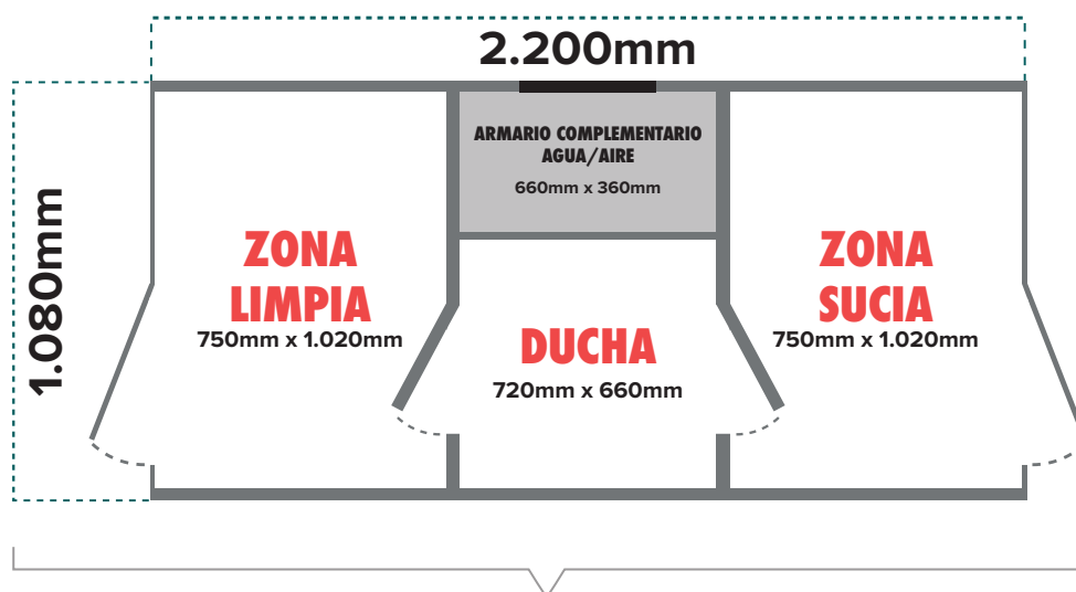
Plano a escala de U.M.D. Modelo: 220/10 F.R.
